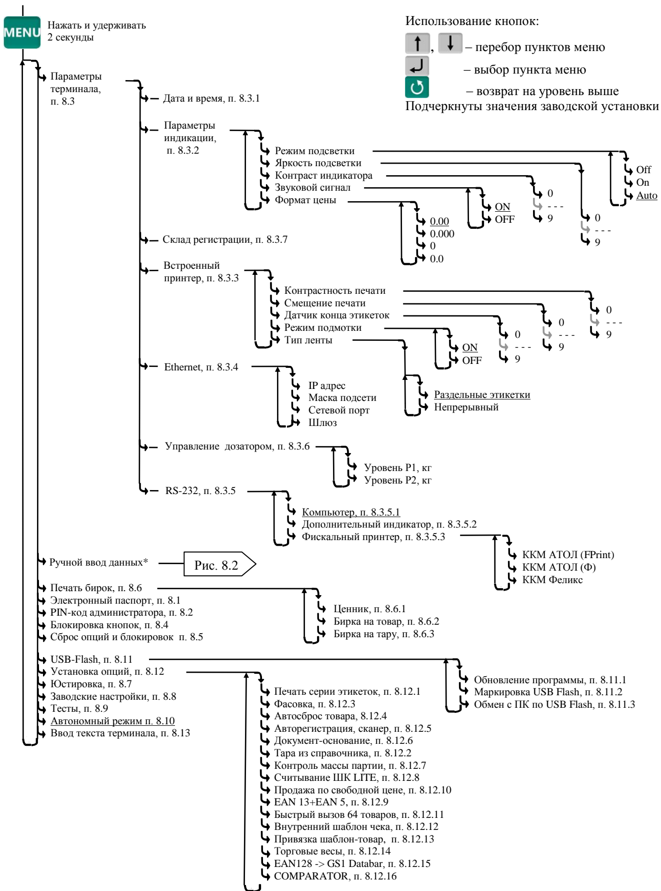
Рис. 8.1 – Структура меню администратора
